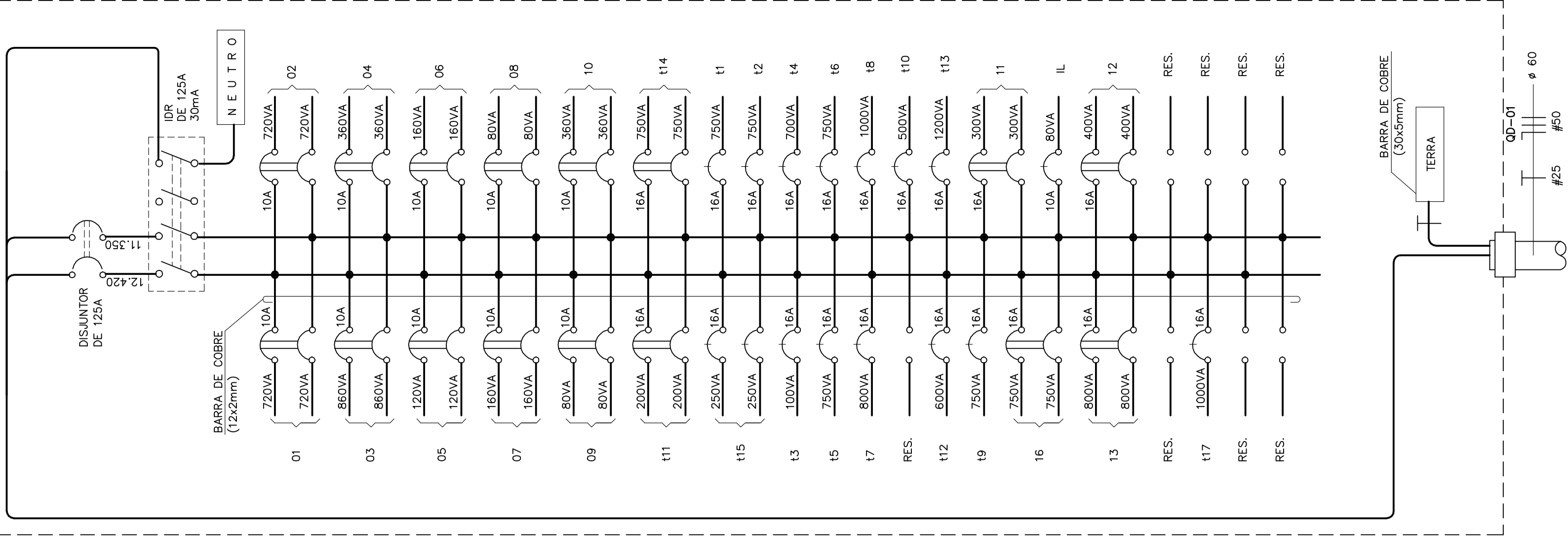
QD-01 (SISTEMA DELTA COM NEUTRO 2F+N) DIMENSÕES APROXIMADAS = 4,22x3,08x17,7m
